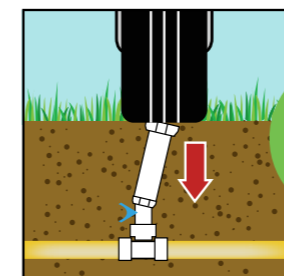
Montage auf Standrohr
