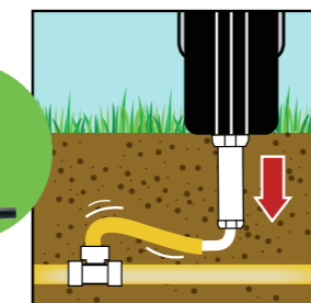
Montage mit SPX-Flex und Verbindungsstücken
